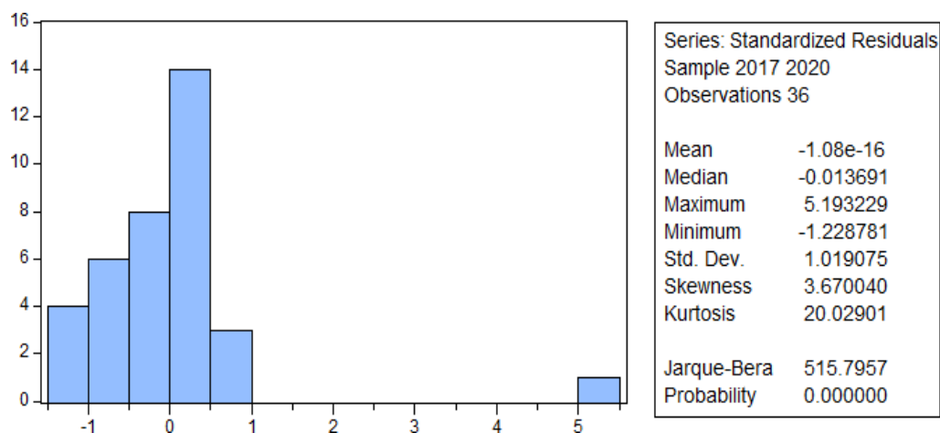
Gambar 4.1 Uji Normalitas
